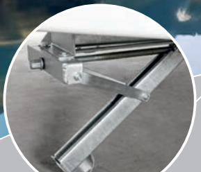
4 Stabilisierungsstützen
